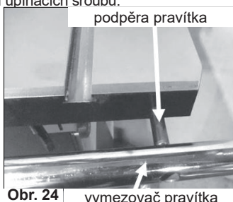
vymezovač pravítka
